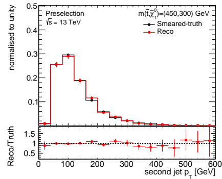
(d) 2 nd leading jet p_T
