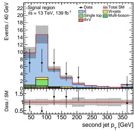
(d) 2 nd leading jet p_T
